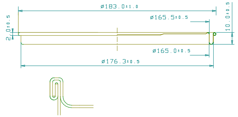
B部(巻き締め)詳細
