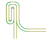
B部(巻き締め)詳細
