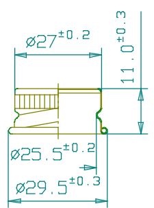
27ネジ蓋
