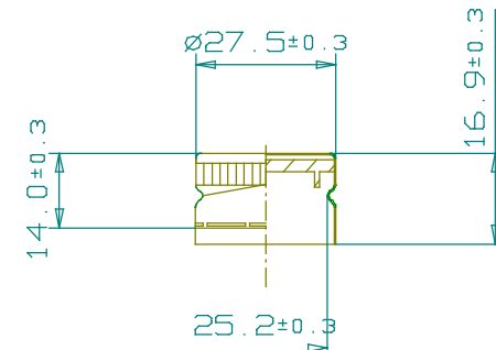
27PPネジ付きキャップ
