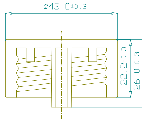
ネジ蓋
