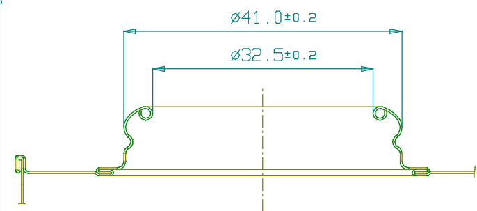
A-A断面(ローヤル詳細尺度1/2)
