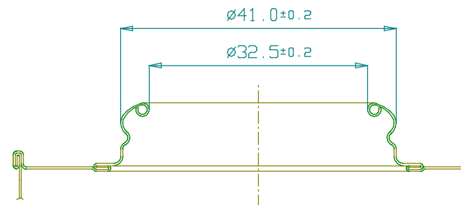
A-A断面(ローヤル詳細尺度1/2)
